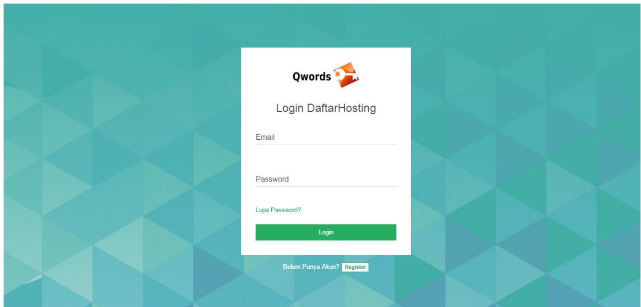
Gambar 3.1 Halaman Login
